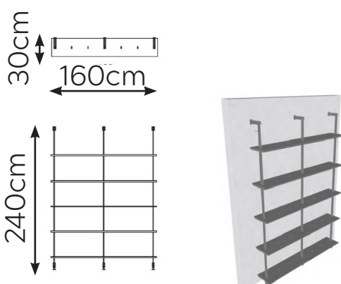
WALL (COMPOSITION 2-001) W: 160cm D: 30cm H: 240cm
