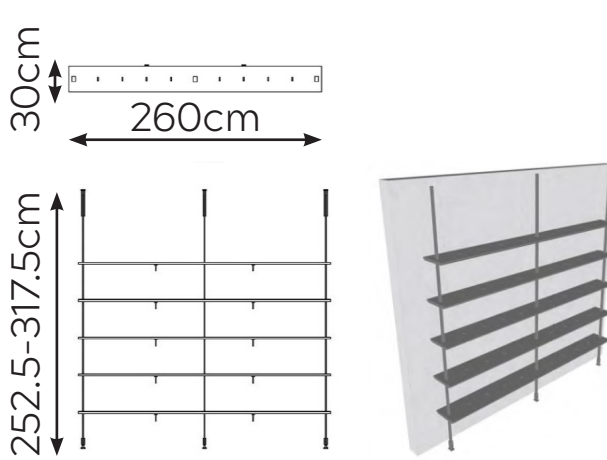
CEILING (COMPOSITION 3-001) W: 260cm D: 30cm H: 252.5-317.5cm
