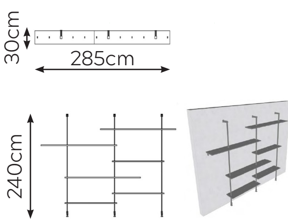
WALL (COMPOSITION 3-004) W: 285cm D: 30cm H: 240cm
