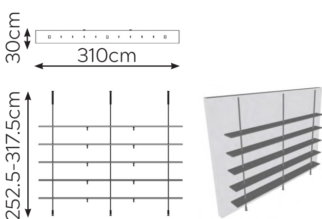
CEILING (COMPOSITION 3-008) W: 310cm D: 30cm H: 252.5-317.5cm
