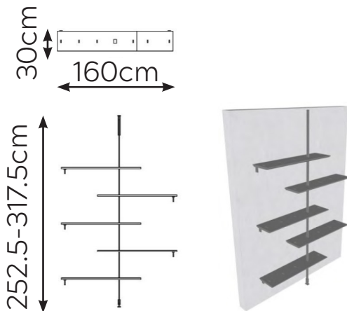
CEILING (COMPOSITION 2-002) W: 160cm D: 30cm H: 252.5-317.5cm
