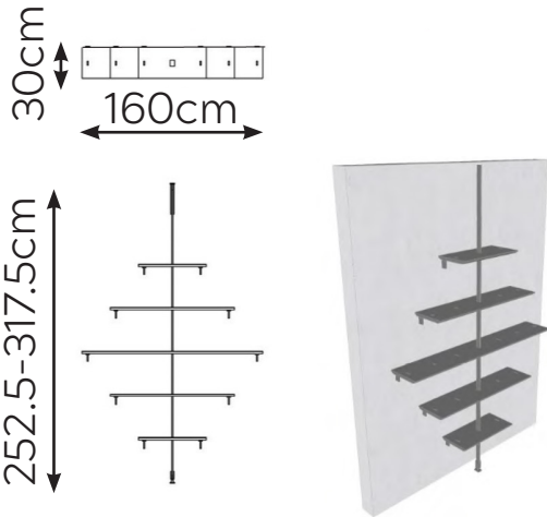
CEILING (COMPOSITION 2-003) W: 160cm D: 30cm H: 252.5-317.5cm
