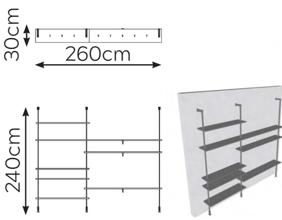
WALL (COMPOSITION 3-003) W: 260cm D: 30cm H: 240cm
