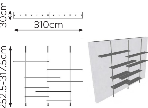
CEILING (COMPOSITION 3-006) W: 310cm D: 30cm H: 252.5-317.5cm
