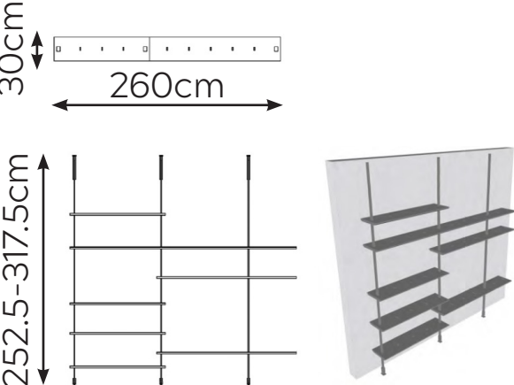
CEILING (COMPOSITION 3-002) W: 260cm D: 30cm H: 252.5-317.5cm
