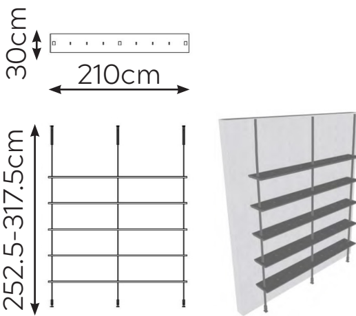
CEILING (COMPOSITION 2-004) W: 210cm D: 30cm H: 252.5-317.5cm
